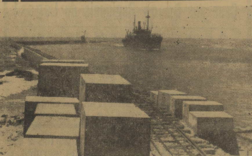
A entrada da barra do porto de Faro-Olhão, agora dotado com 4.500 contos para o prosseguimento dos importantes trabalhos que nele estão sendo realizados. (Vide notícia noutro local).
