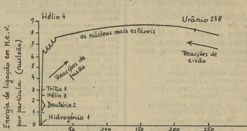
GRÁFICO DA ENERGIA DE LIGAÇÃO DOS DIVERSOS NÚCLEOS
